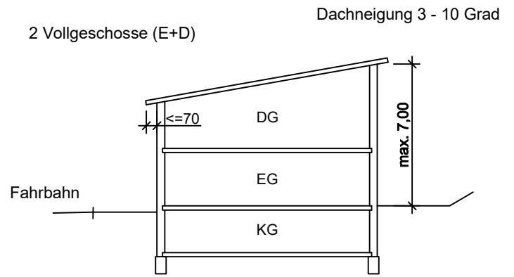
Typ IV Pultdach (zulässig für alle Parzellen)
