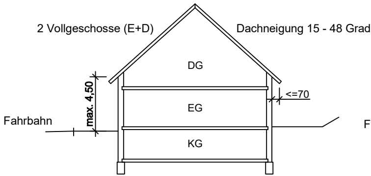
Typ I Satteldach (zulässig für alle Parzellen)
