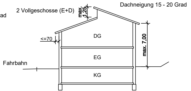
Typ III versetztes Pultdach (zulässig für alle Parzellen)
